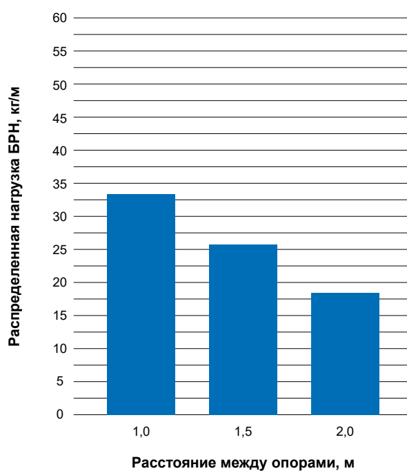
Лоток проволочный ПП4, борт 60 мм
