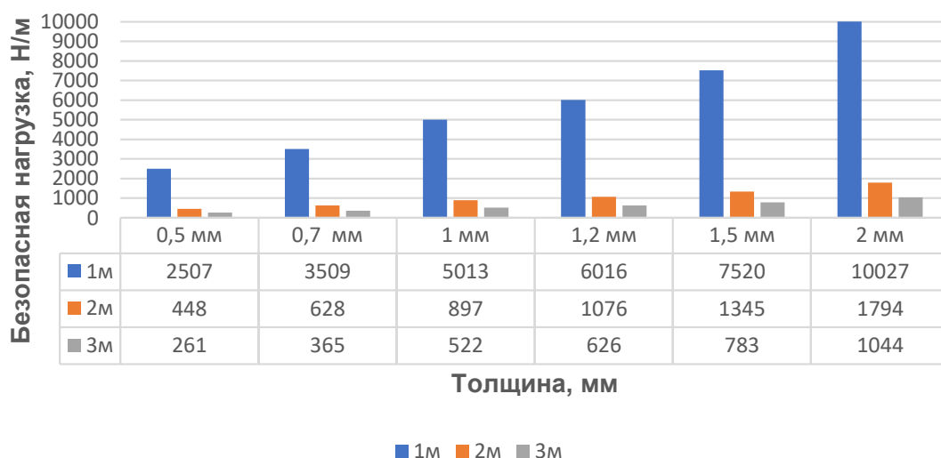
Лоток монтажный ЛП борт 200 мм
