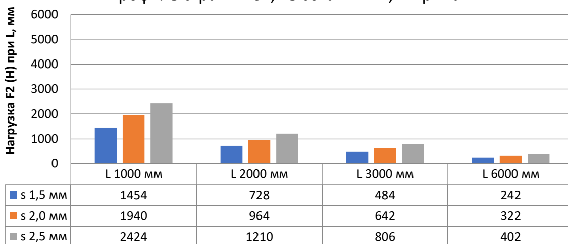
Профиль страт БПС2, высота 42 мм, ширина 41 мм
