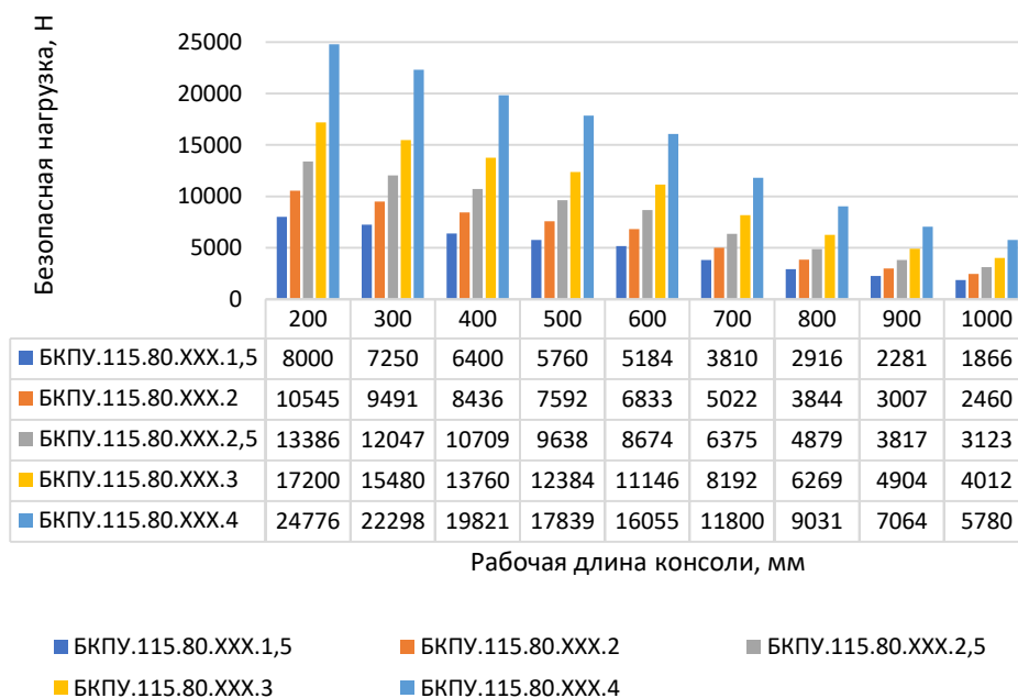
Консоль П - образная усиленная БКПУ, ширина 115 мм, высота 80 мм
