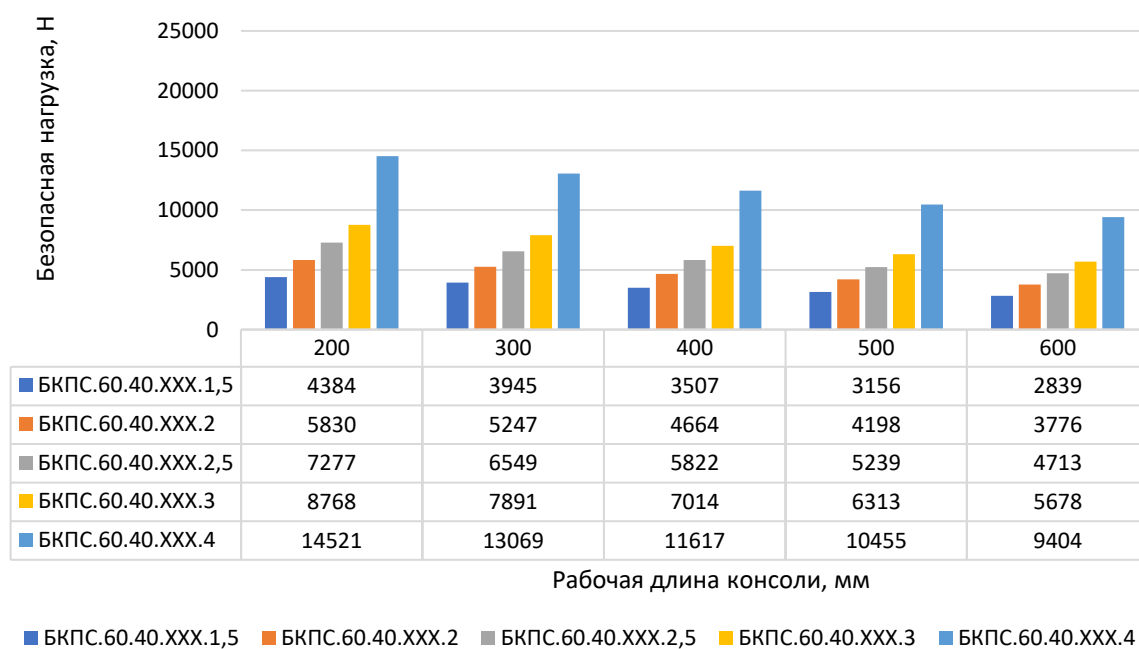
Консоль П - образная средняя БКПС, ширина 60 мм, высота 40 мм
