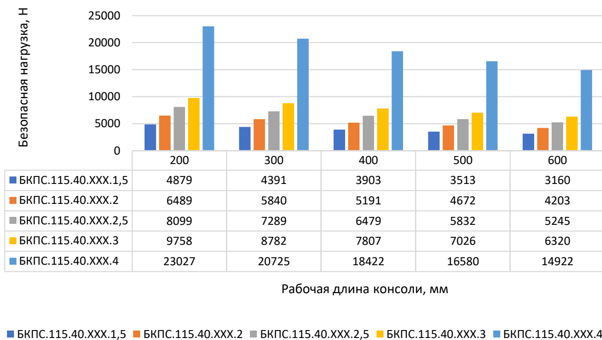
Консоль П - образная средняя БКПС, ширина 115 мм, высота 40 мм
