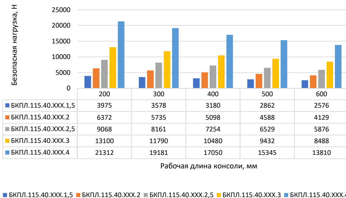
Консоль П - образная легкая БКПЛ, ширина 115 мм, высота 40 мм
