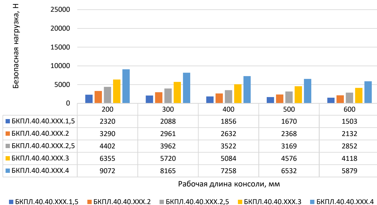
Консоль П - образная легкая БКПЛ, ширина 40 мм, высота 40 мм
