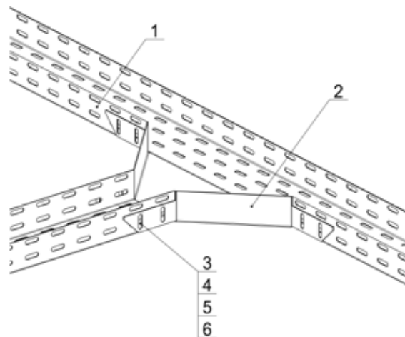
Соединение прямого лотка с ответвительным Изменение трассы для получения отвода
