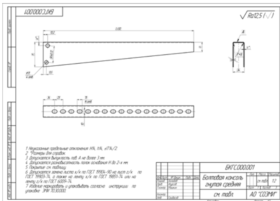
Болтовая консоль гнутая средняя БКГС, ширина 34 мм, высота 75 мм
