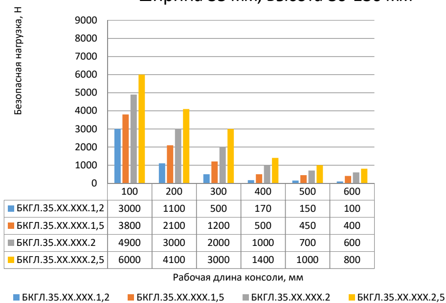
Болтовая консоль гнутая легкая БКГЛ, ширина 35 мм, высота 80-130 мм
