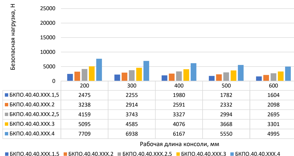
Консоль П - образная облегченная БКПО, ширина 40 мм, высота 40 мм
