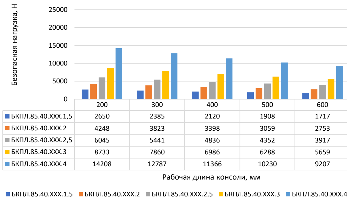
Консоль П - образная легкая БКПЛ, ширина 85 мм, высота 40 мм
