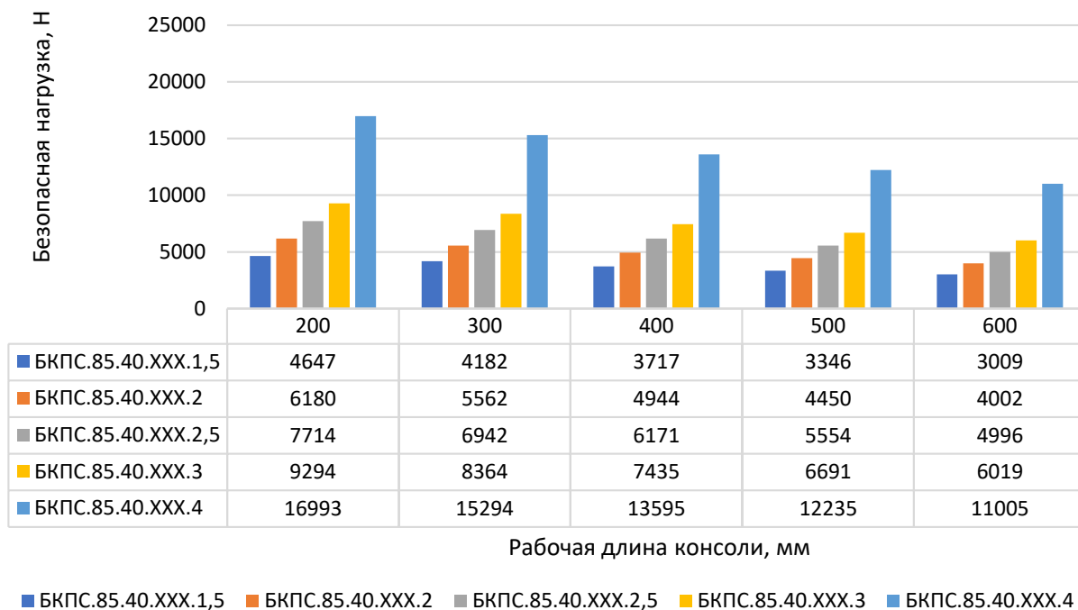
Консоль П - образная средняя БКПС, ширина 85 мм, высота 40 мм
