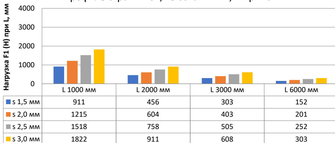
Профиль страт БПС1, высота 41 мм, ширина 41 мм
