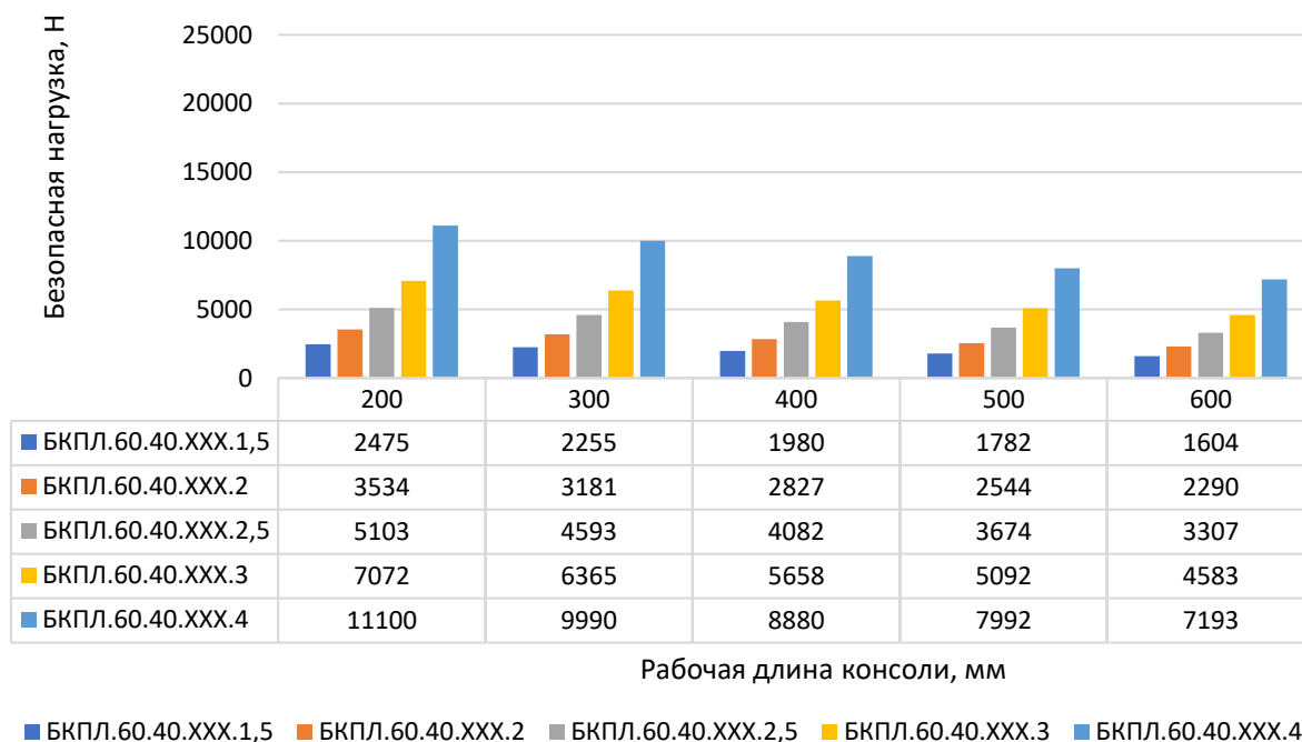
Консоль П - образная легкая БКПЛ, ширина 60 мм, высота 40 мм
