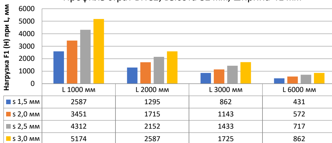
Профиль страт БПС2, высота 82 мм, ширина 41 мм
