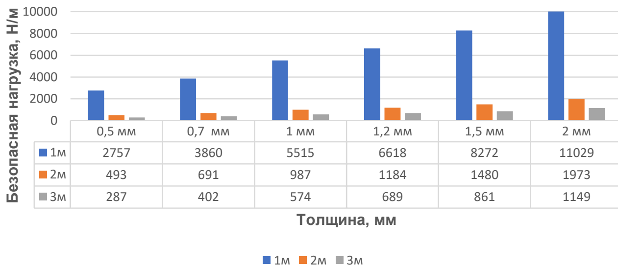
Лоток монтажный ЛПЗ борт 200 мм
