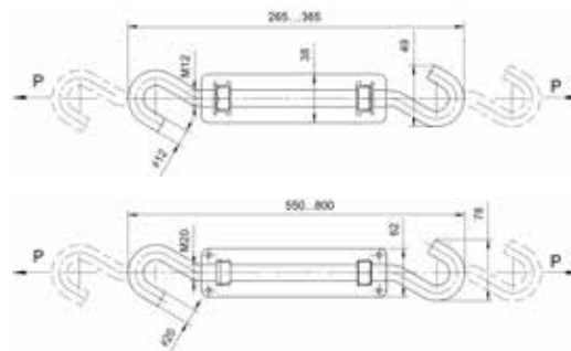
Муфта K804M
