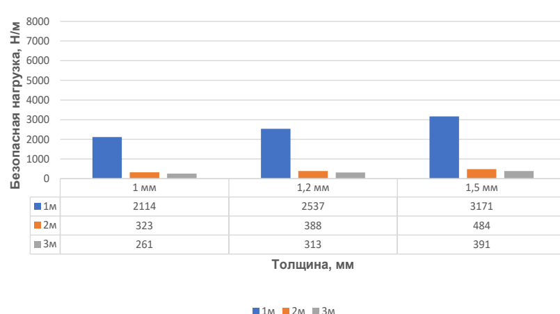
Лоток НЛ 10 борт 24 мм
