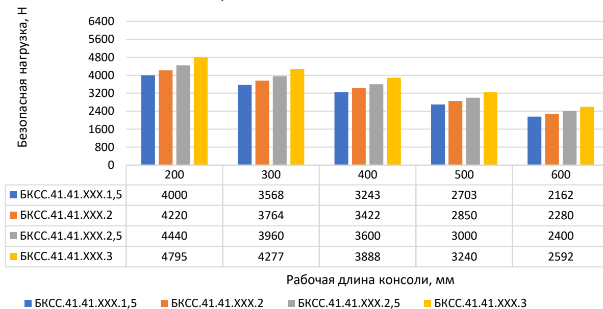
Консоль страт средняя БКСС, ширина 41 мм, высота 41 мм
