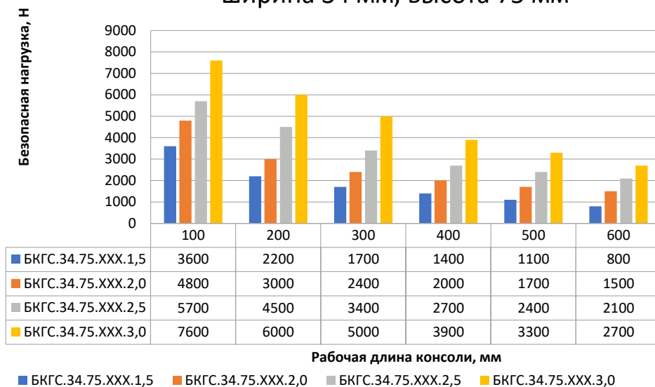
Болтовая консоль гнутая средняя БКГС, ширина 34 мм, высота 75 мм
