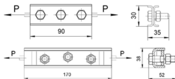
Зажим K676
