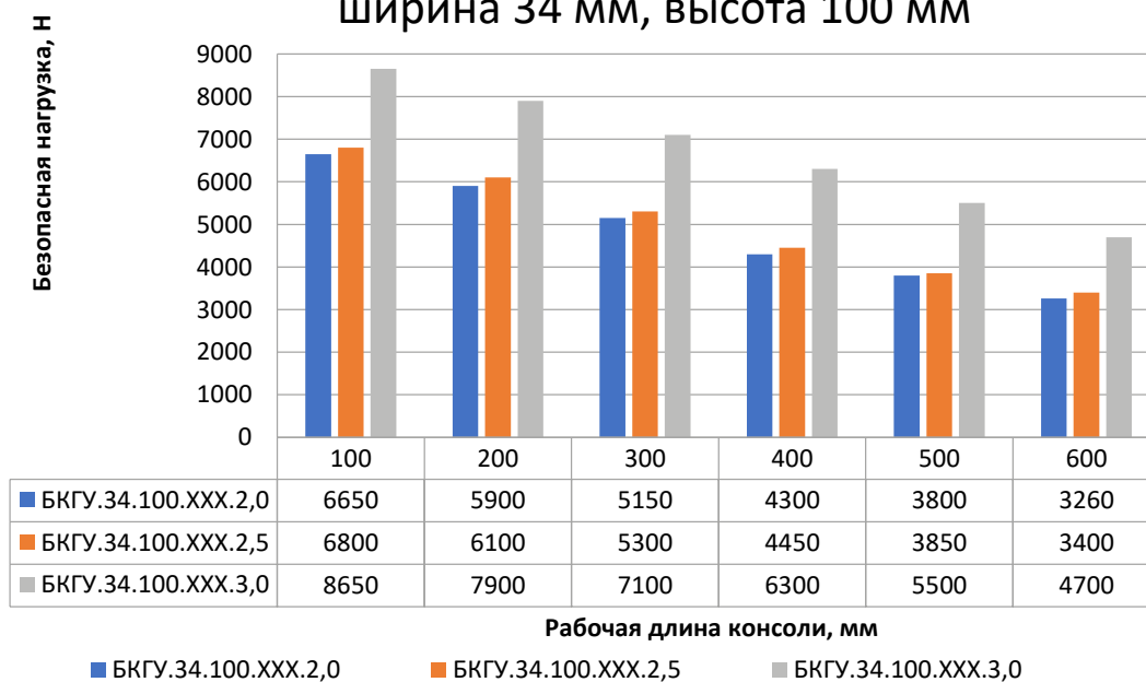
Болтовая консоль гнутая усиленная БКГУ, ширина 34 мм, высота 100 мм
