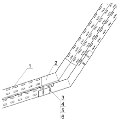
Соединение прямого лотка с угловым Изменение трассы под угол 45° вверх
