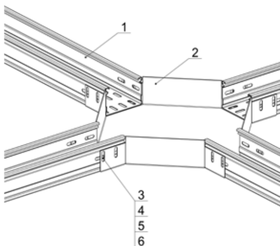
Соединение прямых лотков с крестообразным
