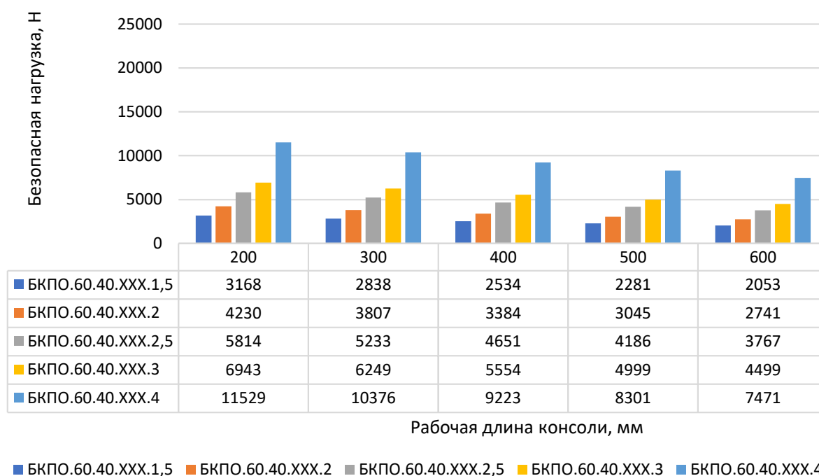
Консоль П - образная облегченная БКПО, ширина 60 мм, высота 40 мм
