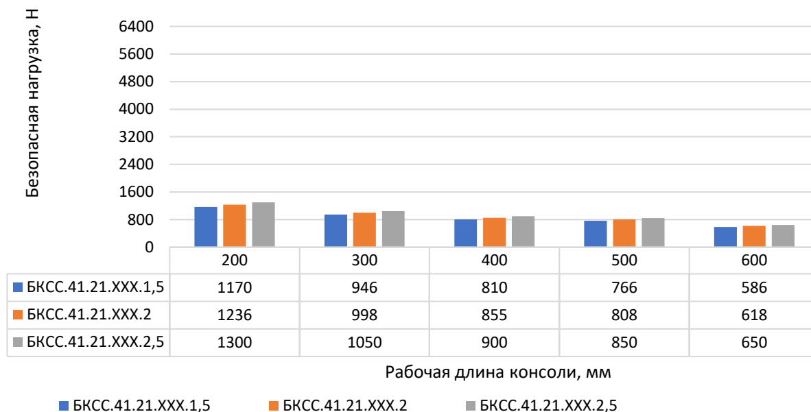
Консоль страт средняя БКСС, ширина 41 мм, высота 21 мм
